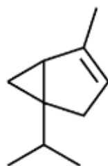
Alpha - thujene
